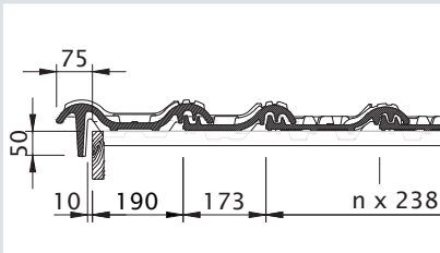
보드가 있는 좌갓기와 설치
