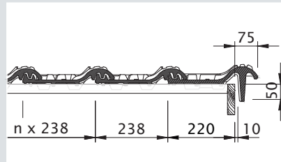
보드가 있는 우갓기와 설치
